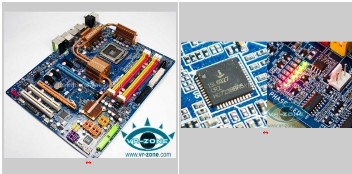
Gigabyte EP35-DS4, ed un particolare della gestione delle fasi d'alimentazione
