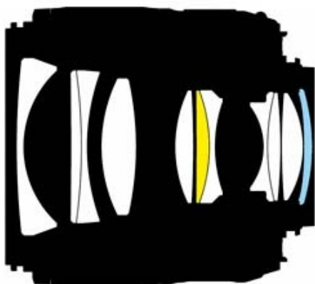
■EDレンズ ■非球面レンズ
